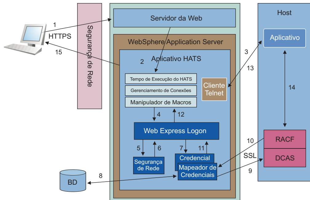
Figura 77. Arquitetura WEL
