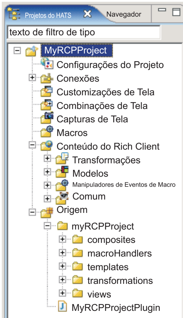
Figura 6. Visualização Projeto do rich client do HATS
