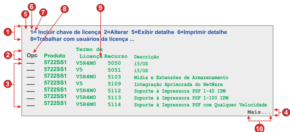
Figura 23. Exemplo de Componente de Subarquivo
