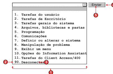
Figura 38. Exemplo de Widget da Lista Drop-down da Lista de Seleção
