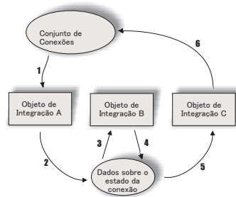
Figura 76. Duração da Conexão com Encadeamento
