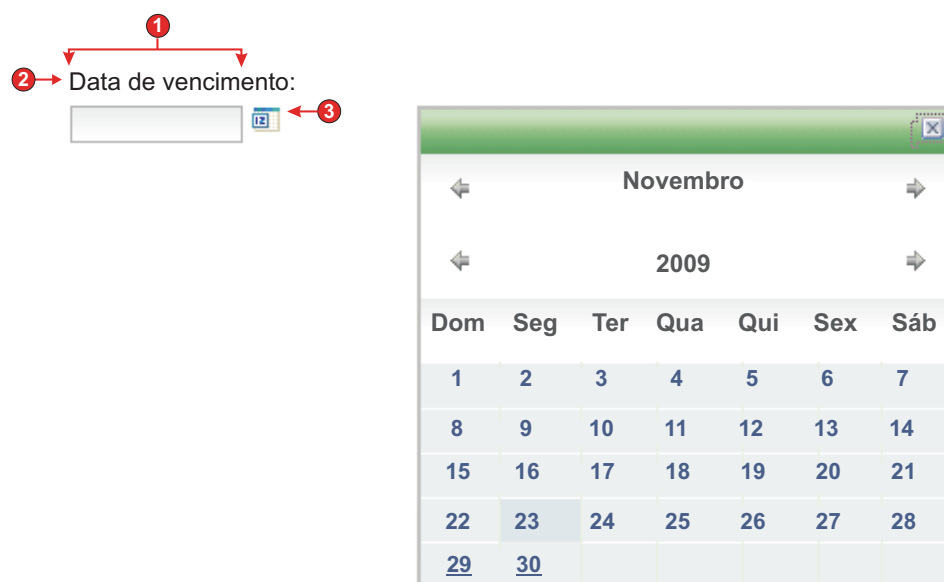
Figura 32. Exemplo de widget de calendário com selecionador de data sequencial
