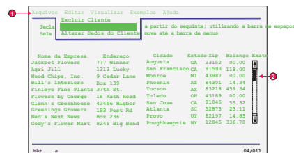
Figura 14. Exemplo de Componentes ENPTUI
